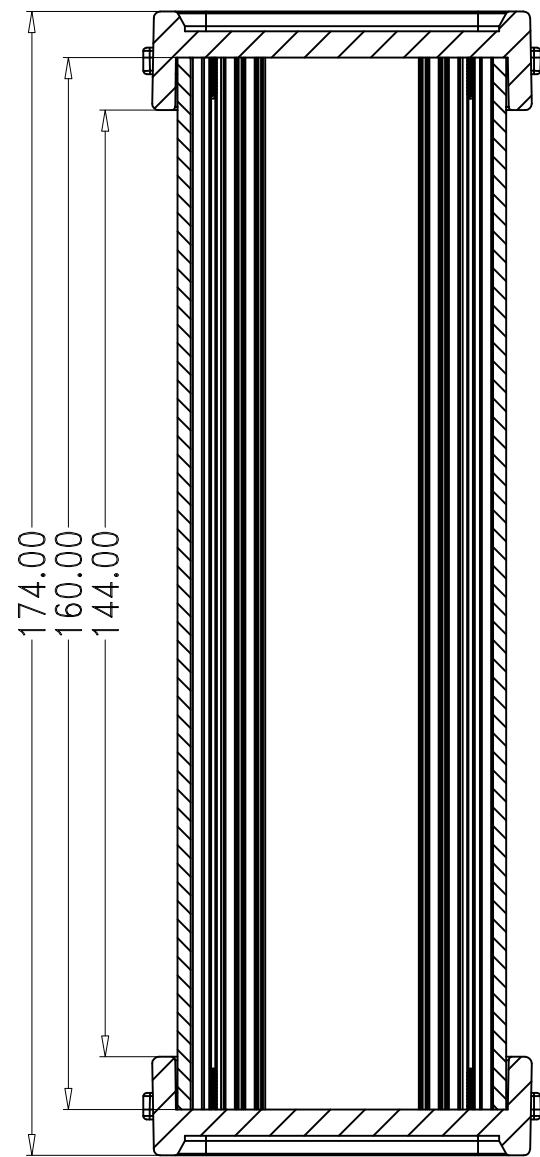
SEC A-A
