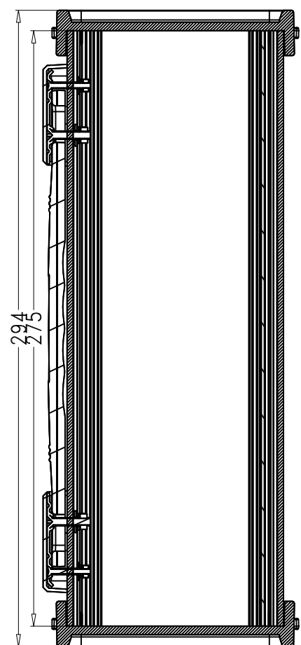
SEC A-A
