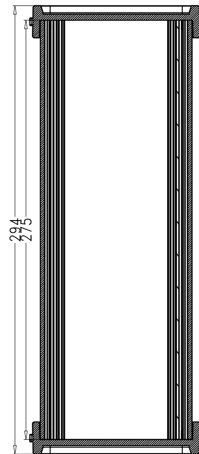
SEC A-A
