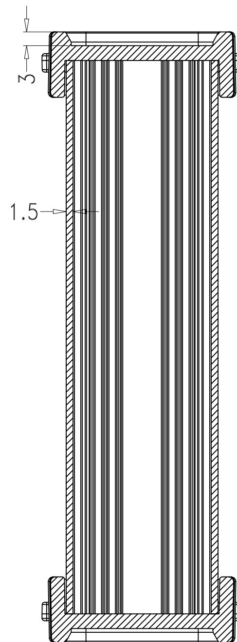
SEC A-A
