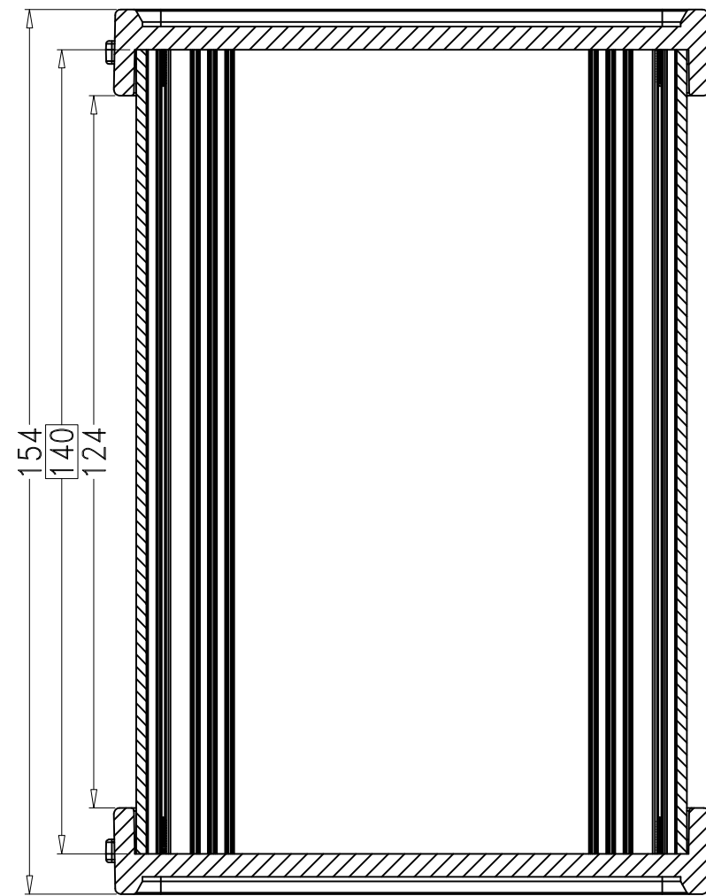
SEC A-A
