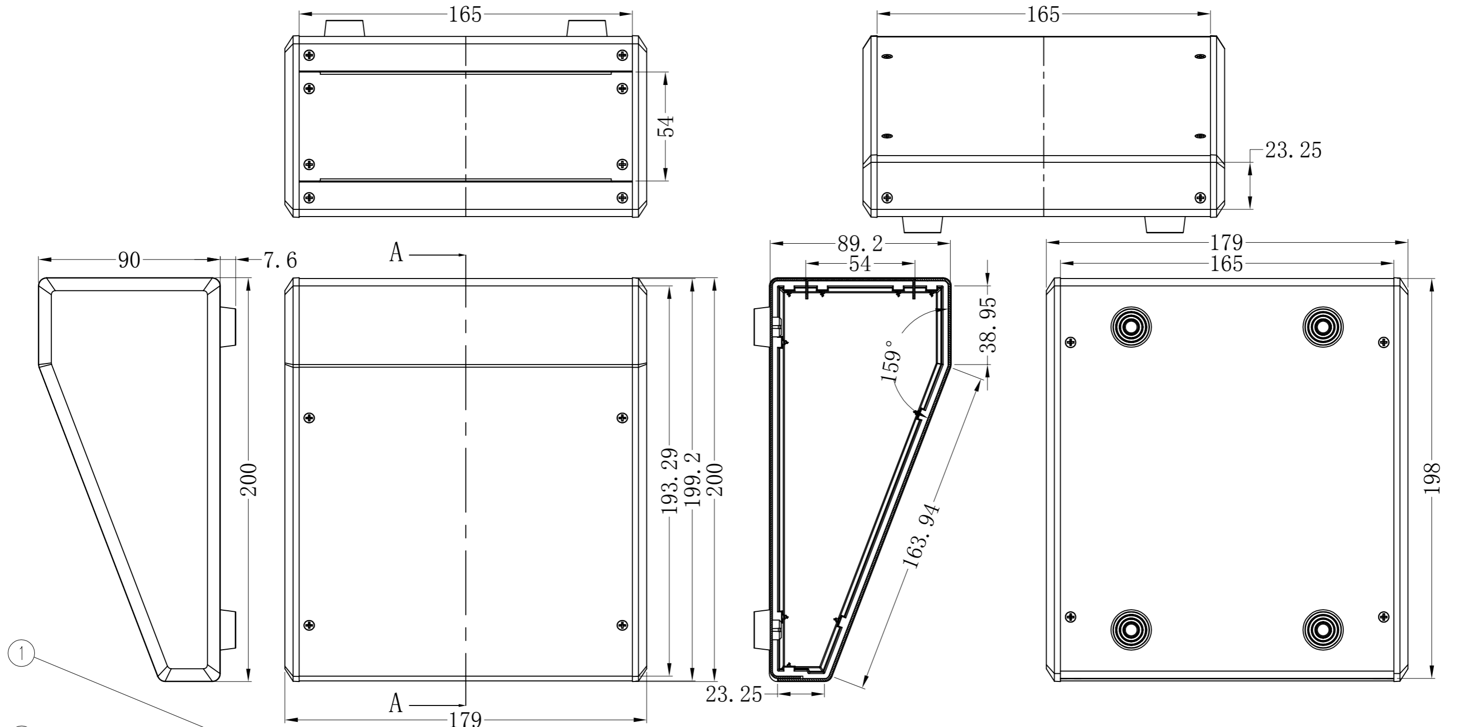
SEC A-A
