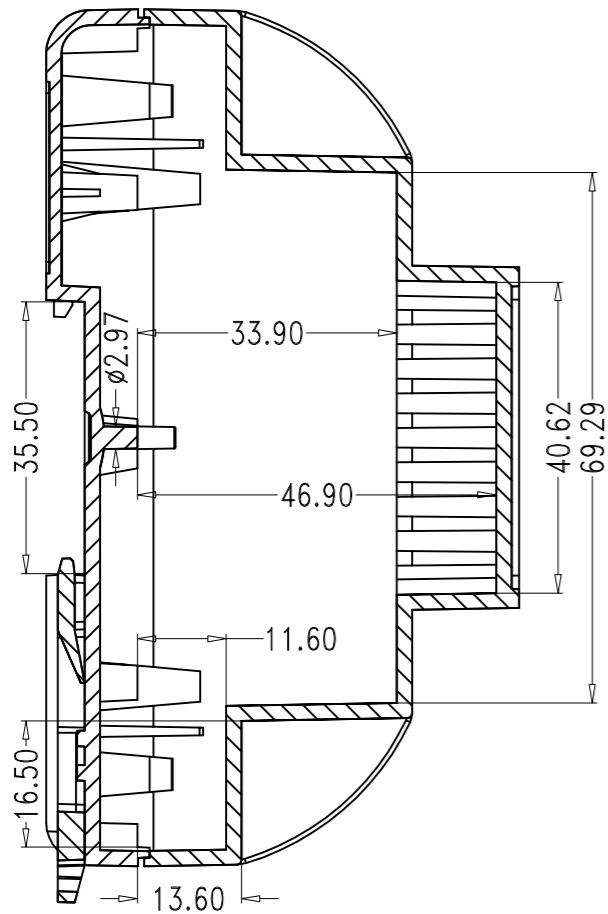
SEC A-A
