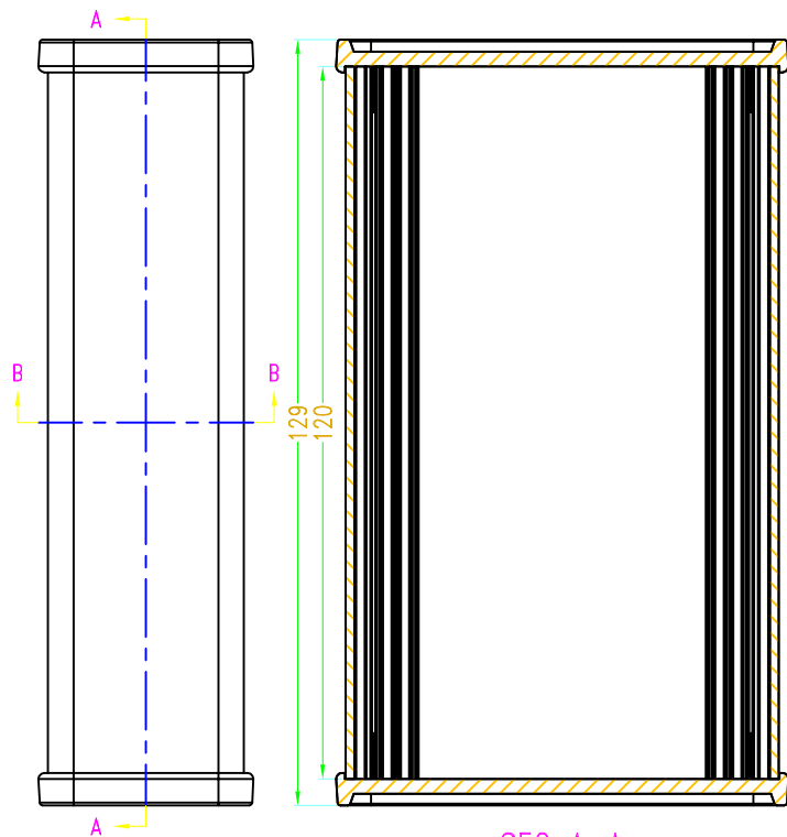
SEC A-A
