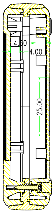
SEC A-A
