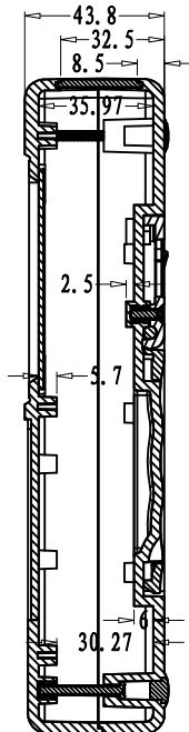
SEC A-A
