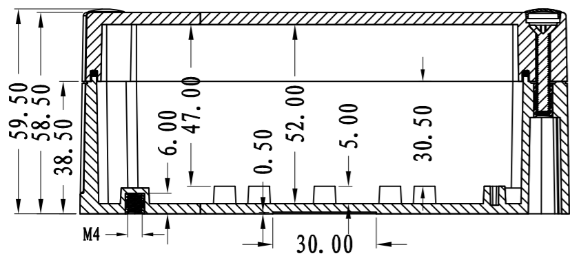
SEC: B-B
