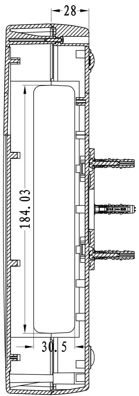
SEC A-A
