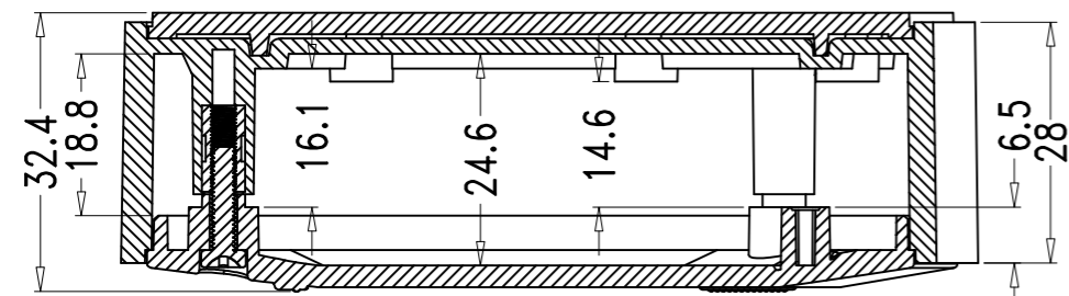
SEC A-A
