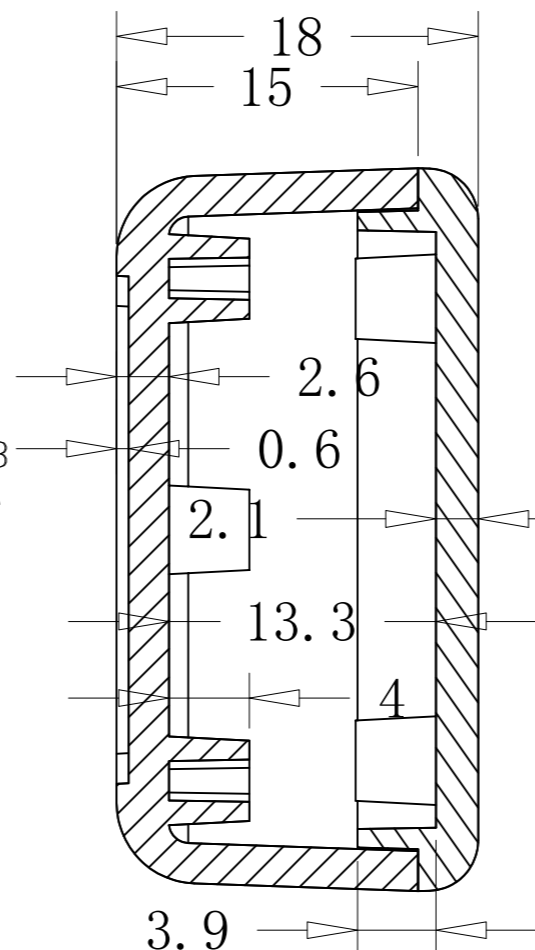
SEC A-A
