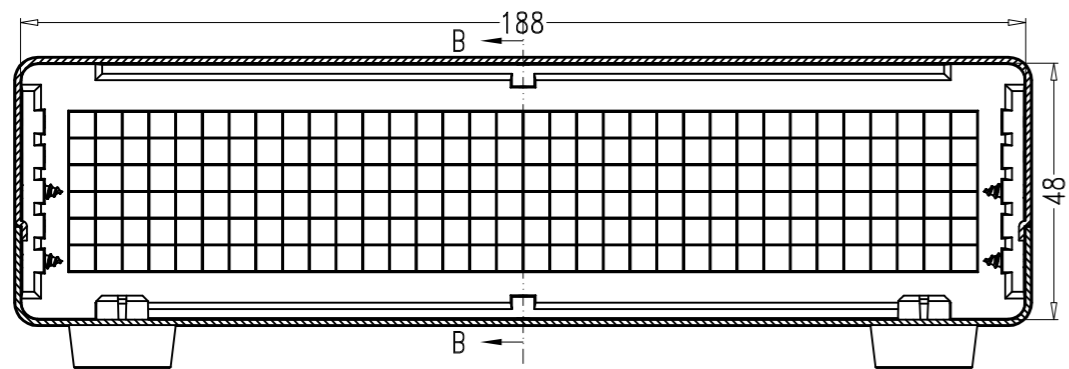
SEC A-A
