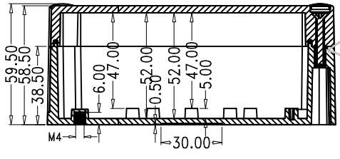
SEC: B-B
