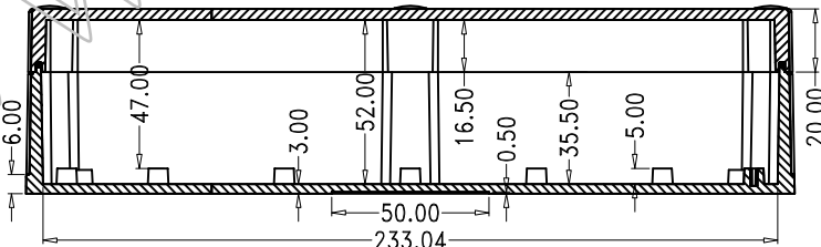
SEC: A-A
