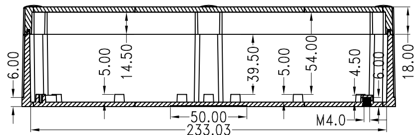
SEC: B-B
