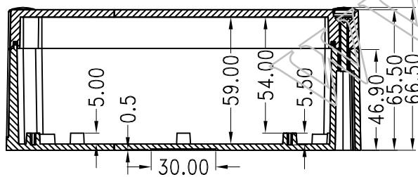
SEC: A-A
