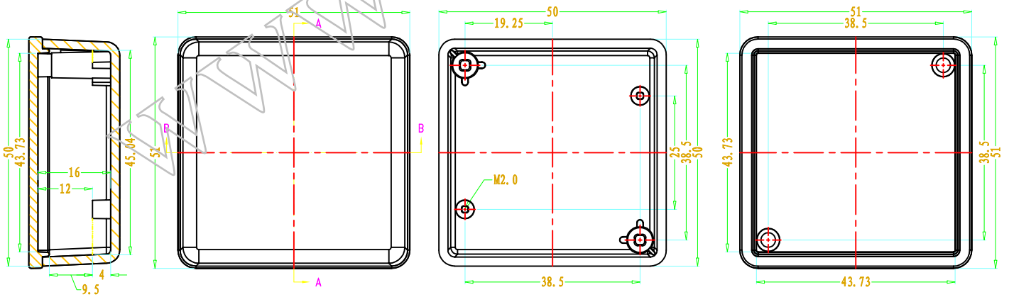
SEC A-A
