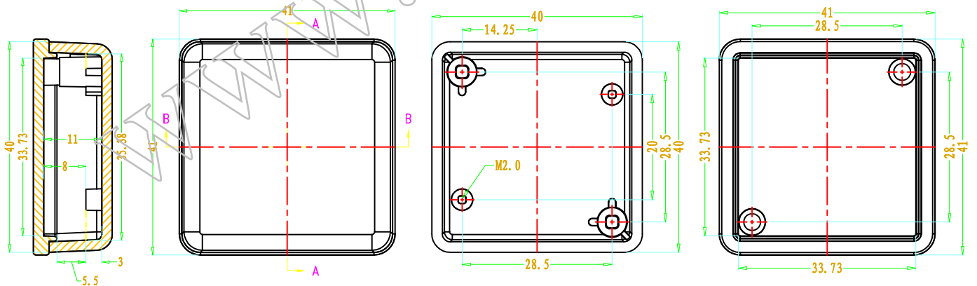
SEC A-A
